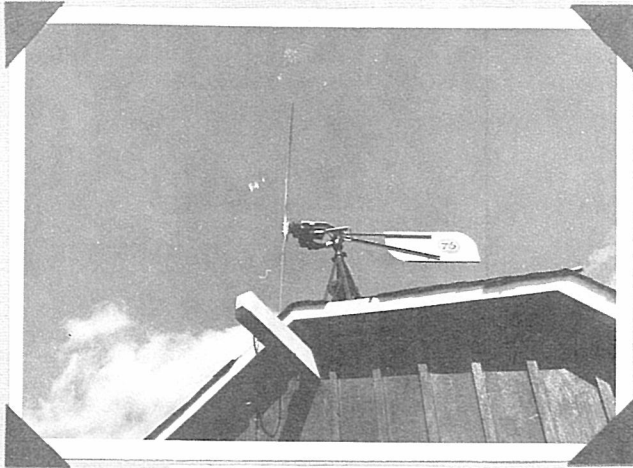
PHOTO 8. Delco 200 Watt - 12 Volt
